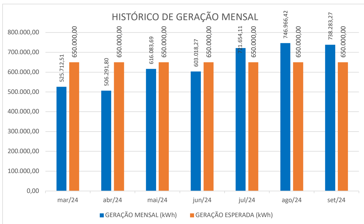
Gráfico 4 - Histórico de geração mensal do segundo ano de operação
