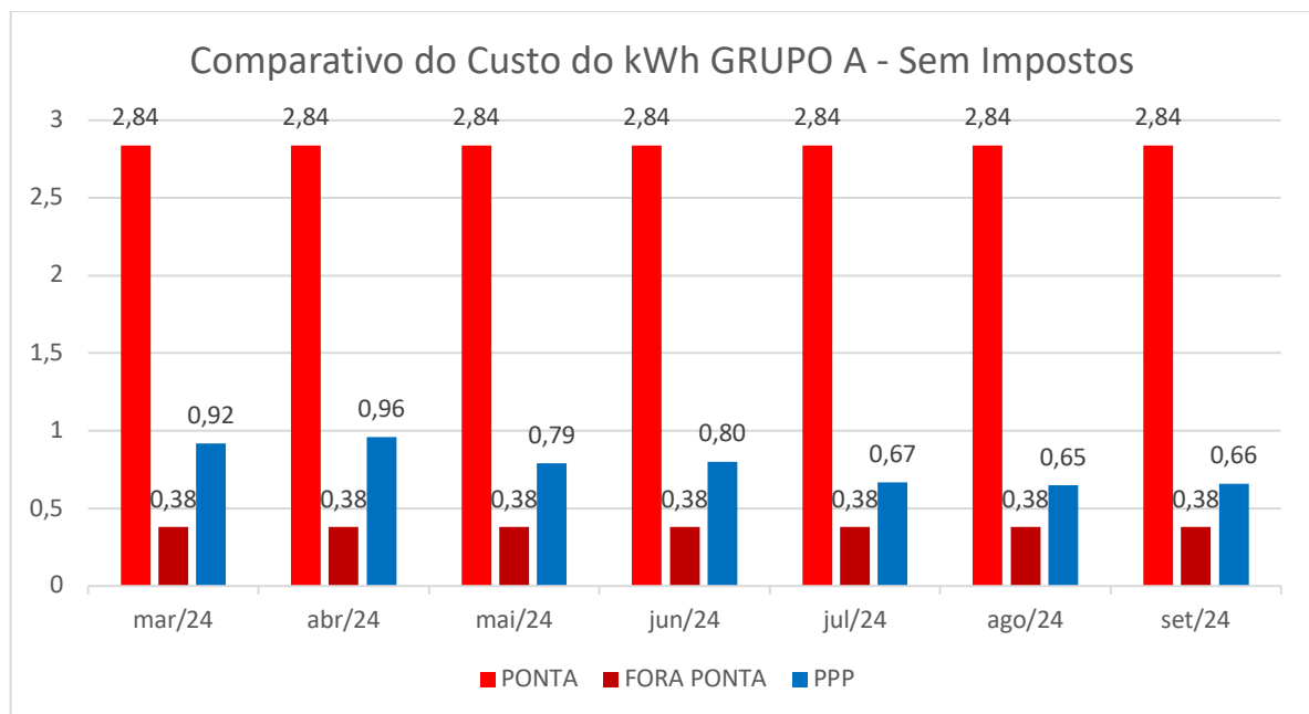
Gráfico 7 - Comparativo dos custos de energia do ACR GRUPO A e da PPP
