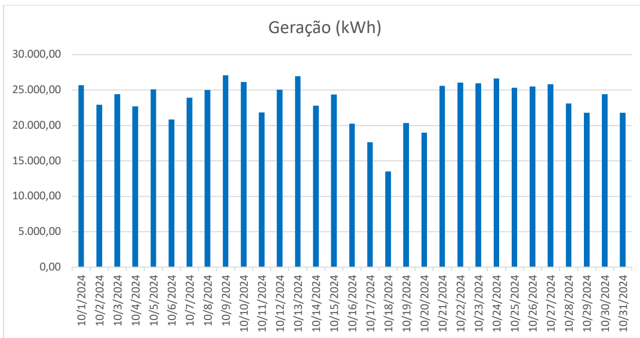
Gráfico 2 - Geração de energia no mês de outubro
