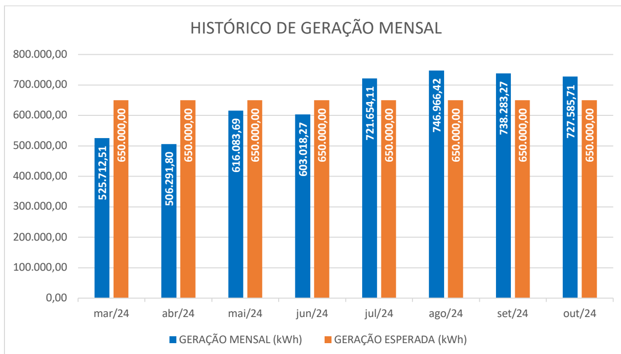
Gráfico 4 - Histórico de geração mensal do segundo ano de operação
