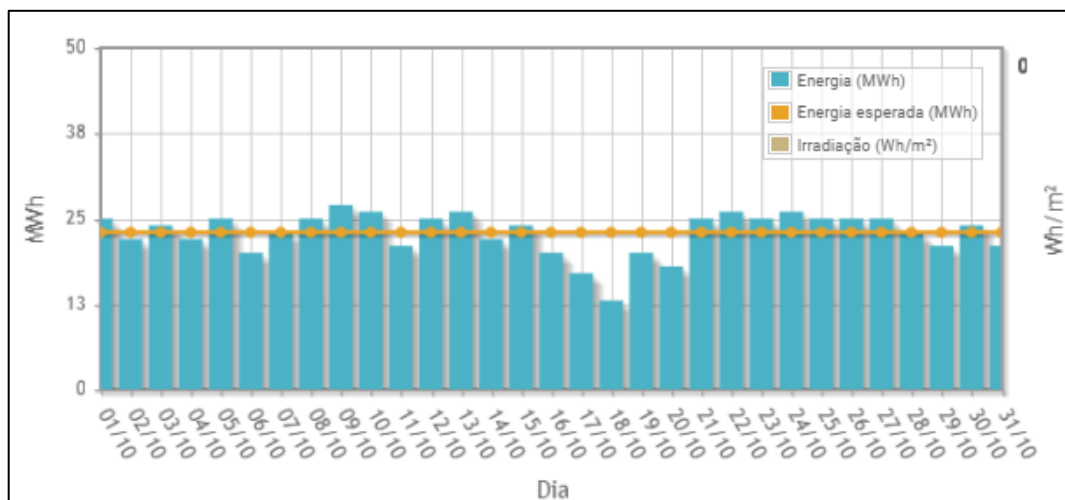
Gráfico 3 - Gráfico de geração fornecido pelo SCADA
