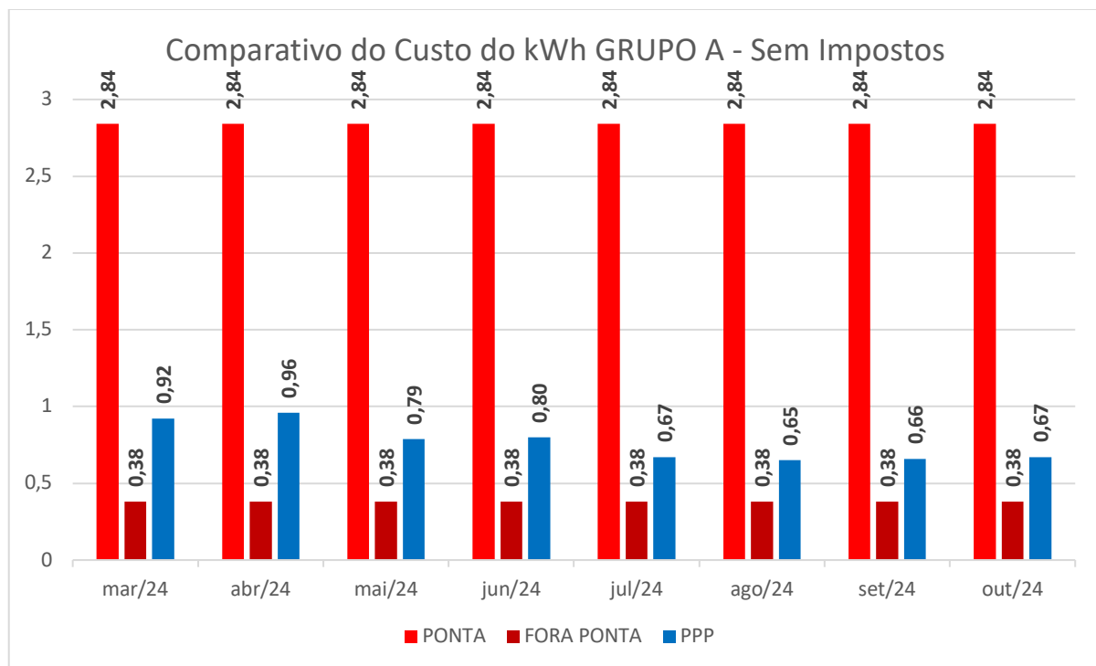
Gráfico 7 - Comparativo dos custos de energia do ACR GRUPO A e da PPP
