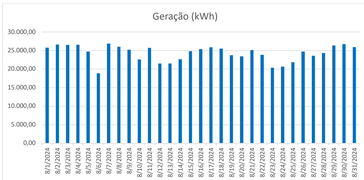
Gráfico 2 - Geração de energia no mês de agosto
