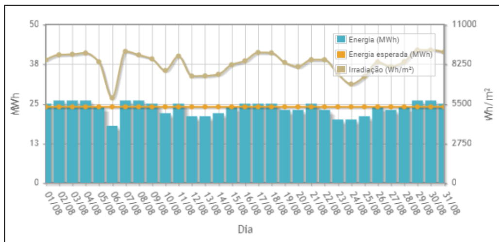
Gráfico 3 - Geração de energia no mês de agosto
