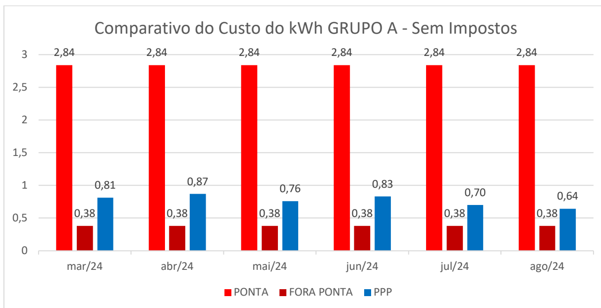
Gráfico 7 - Comparativo do custo do kWh entre o projeto de PPP e o Grupo A (sem imposto)
