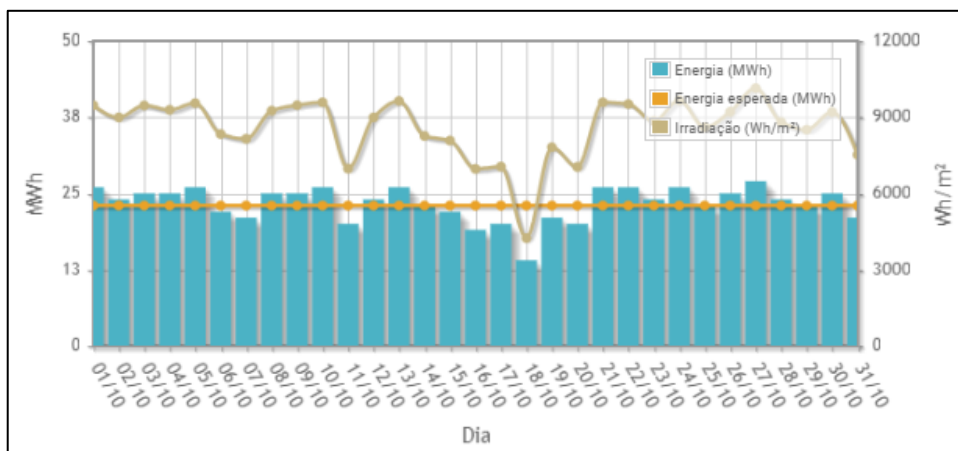
Gráfico 3 - Geração de energia no mês de outubro
