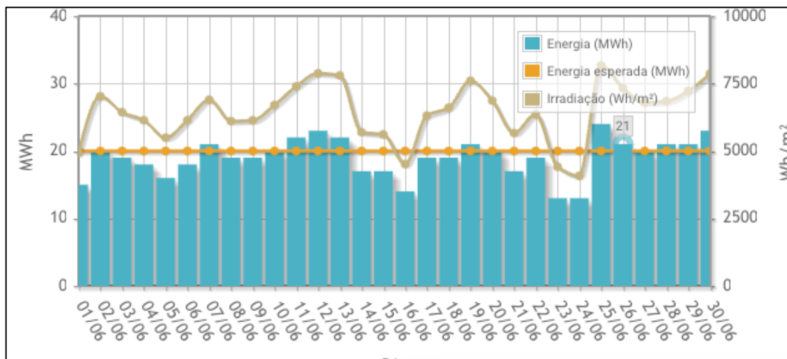
Gráfico 3 - Geração de energia no mês de Junho
