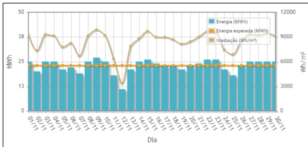
Gráfico 3 - Geração de energia no mês de novembro
