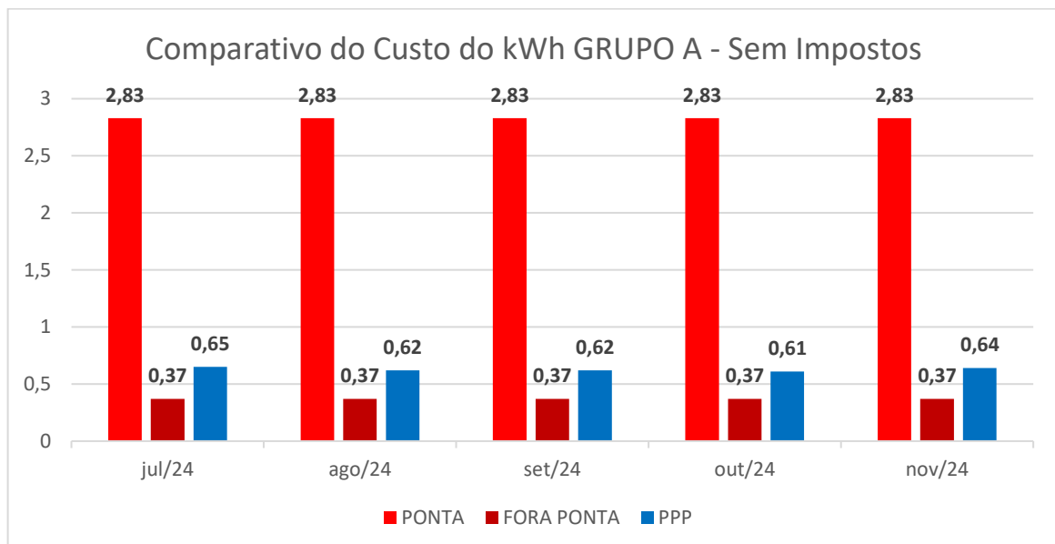
Gráfico 8 - Comparativo do custo do kWh com a trafica do Grupo A (sem imposto)
