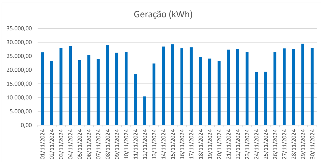
Gráfico 3 - Geração diária das usinas
