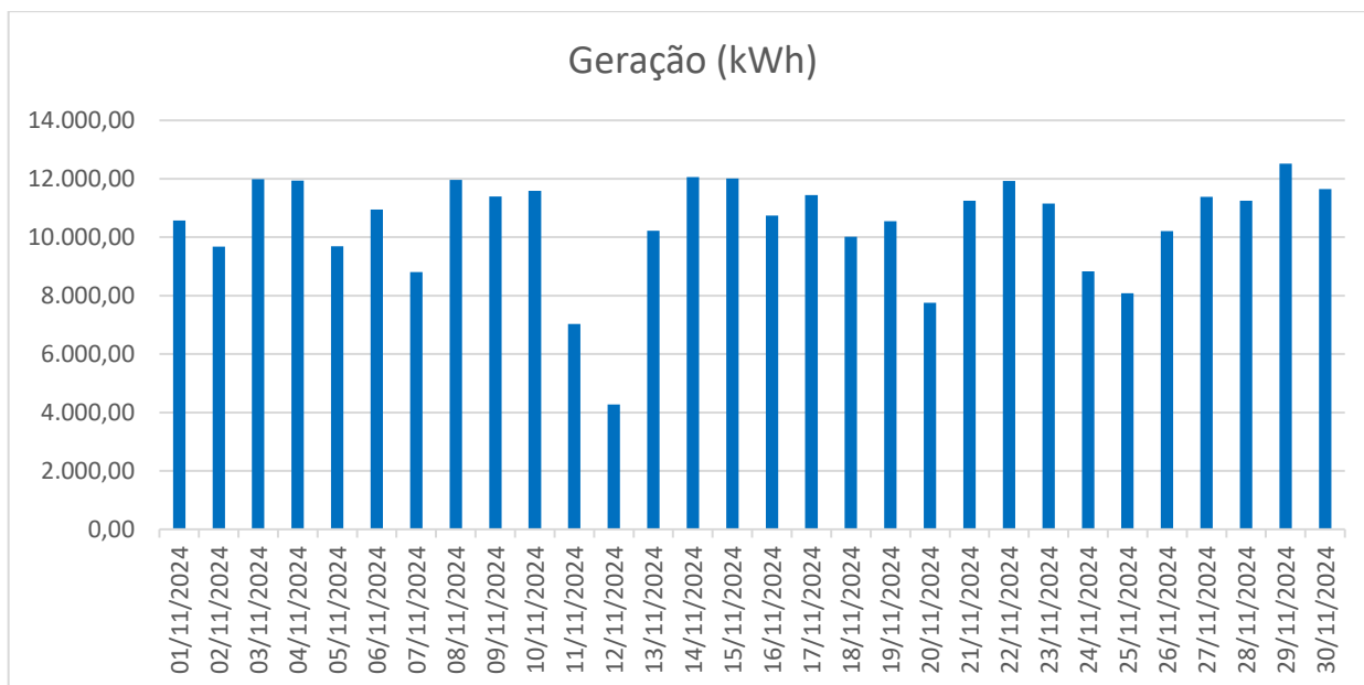
Gráfico 1 - Geração diária da GD Nova Longá
