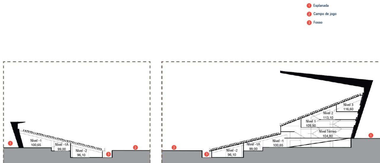
Figura 2 Corte Lateral
