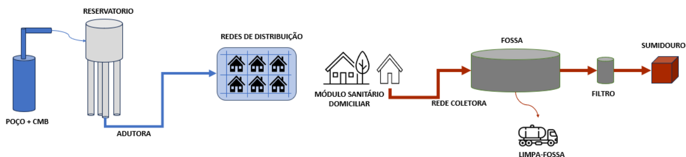
Figura 3 - Diagrama para solução agrupada sugerida para economias rurais dispersas.
