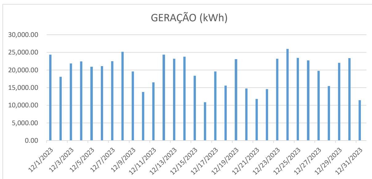
Gráfico 2 - Geração de energia no mês de dezembro
