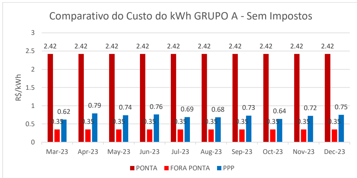
Gráfico 7 - Comparativo dos custos de energia do ACR GRUPO A e da PPP
