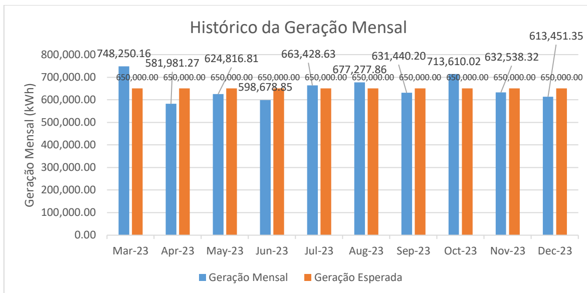
Gráfico 4 - Histórico de geração mensal de 2023
