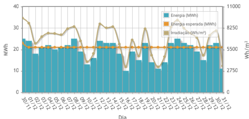
Gráfico 3 - Gráfico de geração fornecido pelo SCADA
