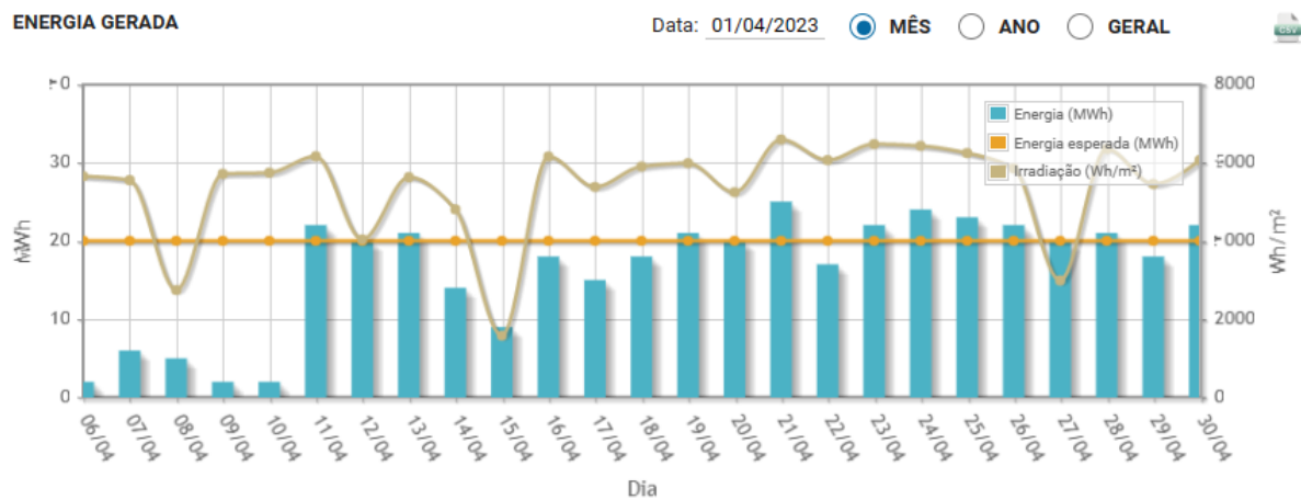
Figura 5 - Gráfico de geração fornecido pelo SCADA
