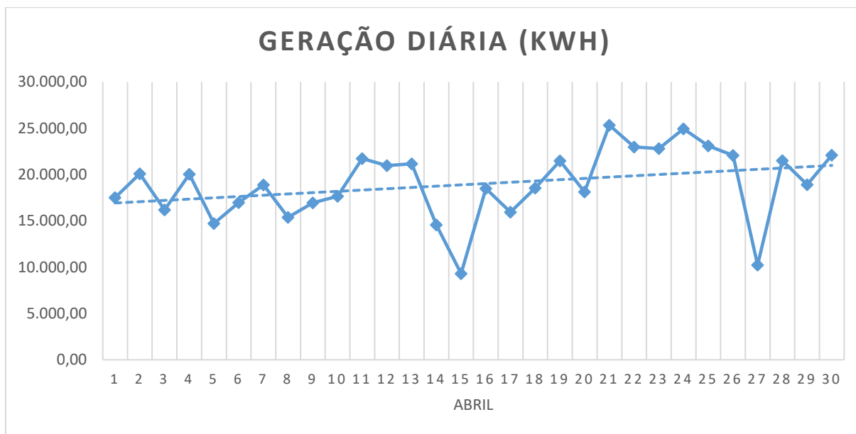
Figura 4 - Geração diária dos inversores
