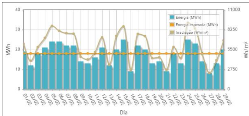
Gráfico 3 - Geração de energia no mês de Fevereiro
