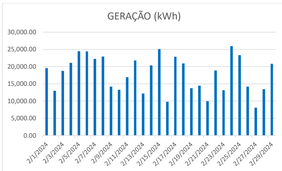
Gráfico 2 - Geração de energia no mês de Fevereiro
