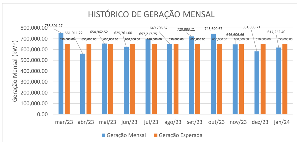
Gráfico 4 - Histórico de geração mensal de 2023
