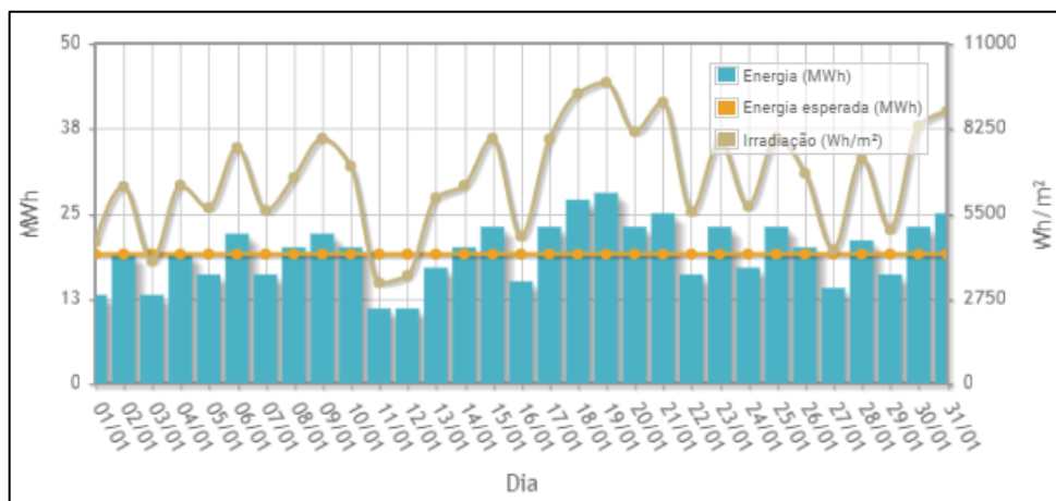
Gráfico 3 - Geração de energia no mês de Janeiro
