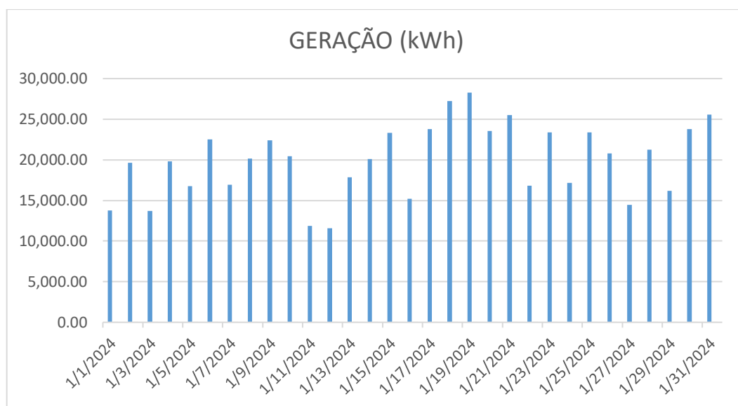
Gráfico 2 - Geração de energia no mês de Janeiro
