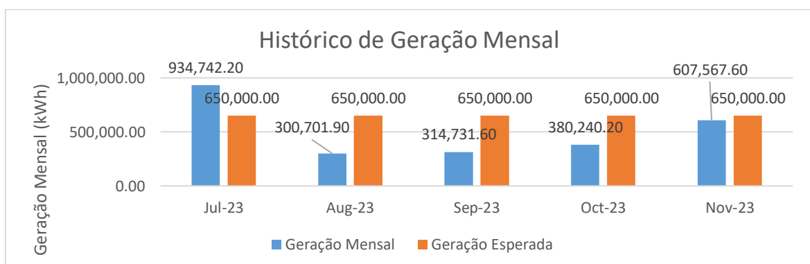
Gráfico 4 - Comparativo da energia gerada com a esperada conforme o EVTEA
