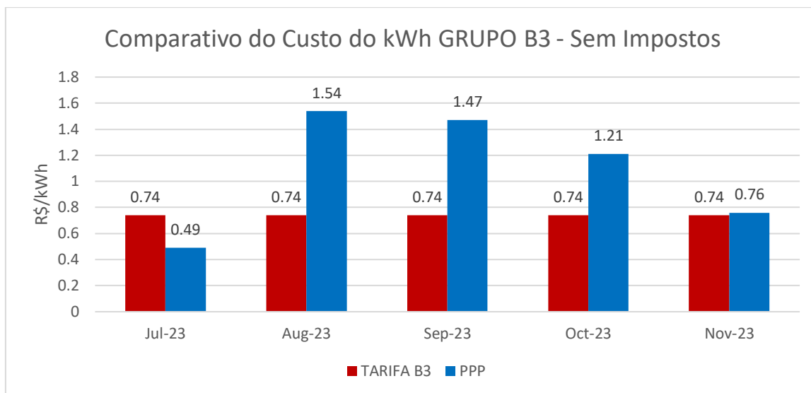
Gráfico 8 - Comparativo do custo do kWh com a trafica do Grupo B (sem imposto)
