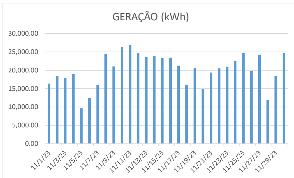
Gráfico 3 - Geração diária das usinas
