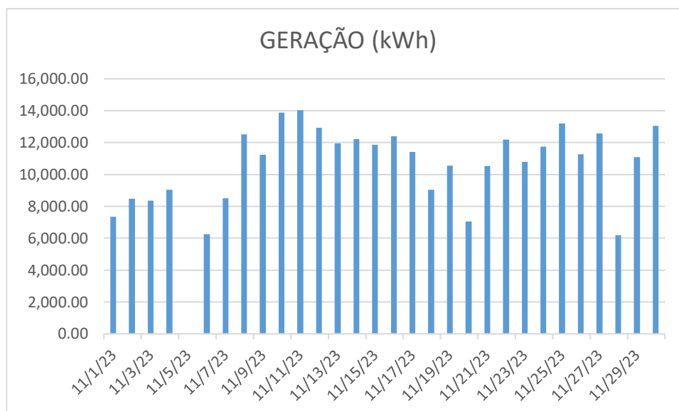
Gráfico 2 - Geração diária da GD Longá
