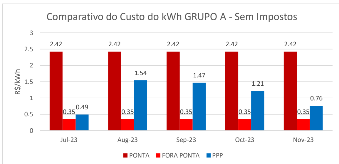
Gráfico 7 - Comparativo do custo do kWh com a tarifa do Grupo A (sem imposto)
