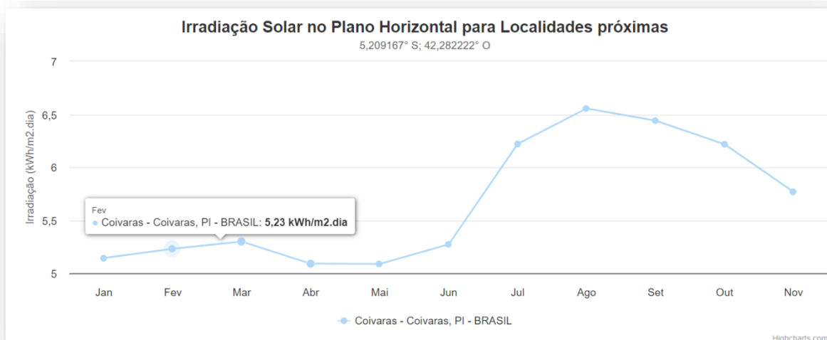
Gráfico 7 - Gráfico da irradiância solar incidente no município de Coivaras
