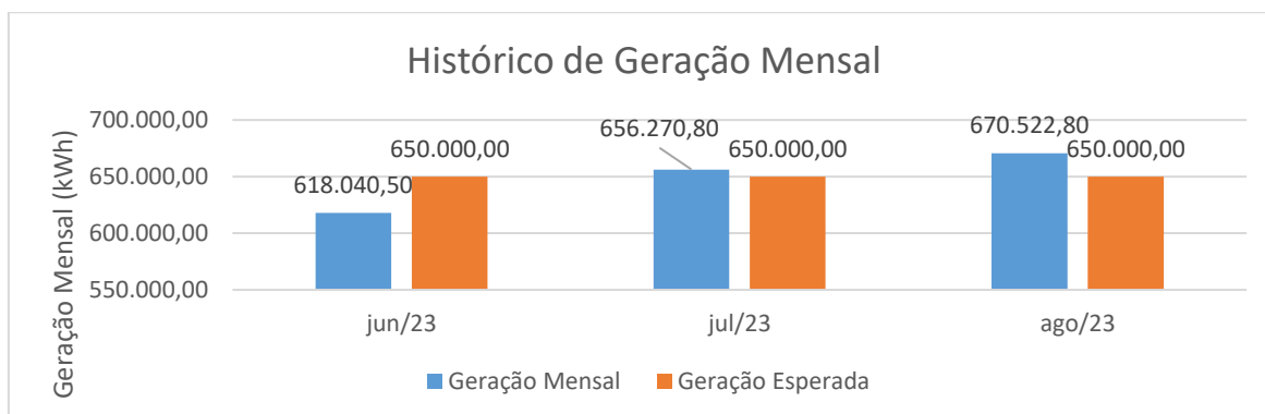
Gráfico 8 - Comparativo da energia gerada com a esperada conforme o EVTEA
