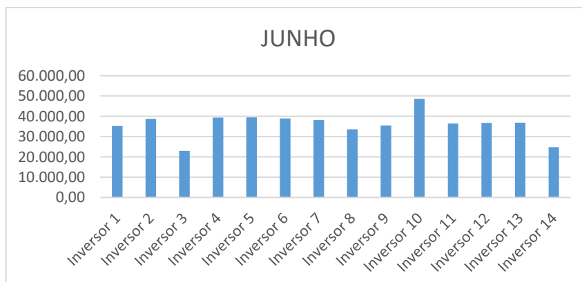
Gráfico 3 - Geração de junho com base nos dados dos inversores
