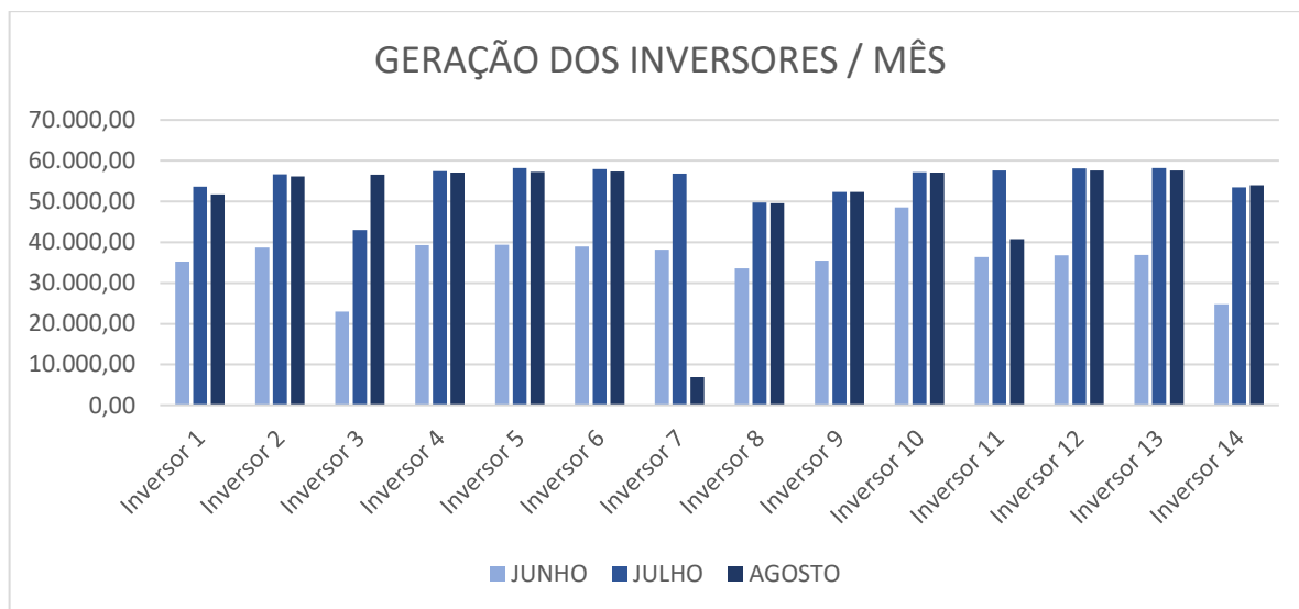
Gráfico 6 - Comparativo mensal da geração de energia de cada inversor
