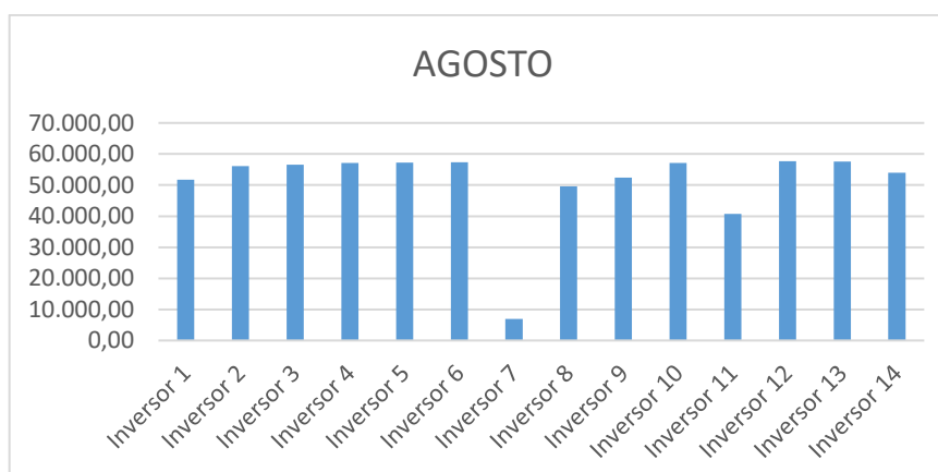
Gráfico 5 - Geração de agosto com base nos dados dos inversores
