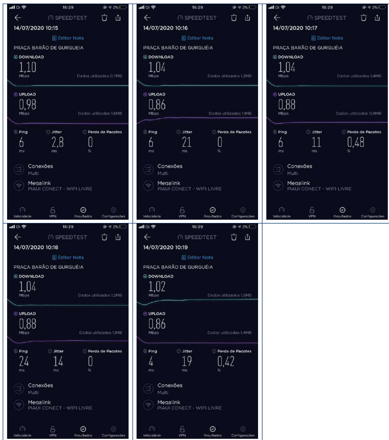
Figura 89 – Aferição da Velocidade do PAP Praça Barão de Gurguéia - Teresina
