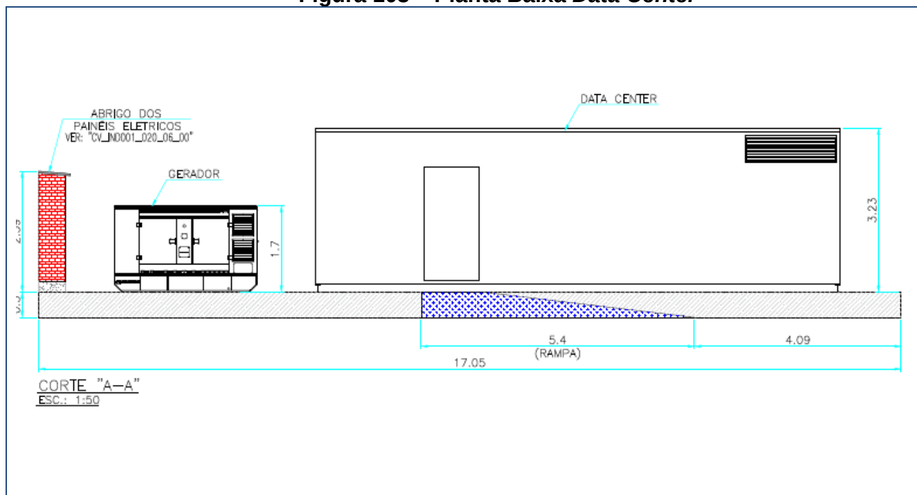
Figura 103 – Planta Baixa Data Center
