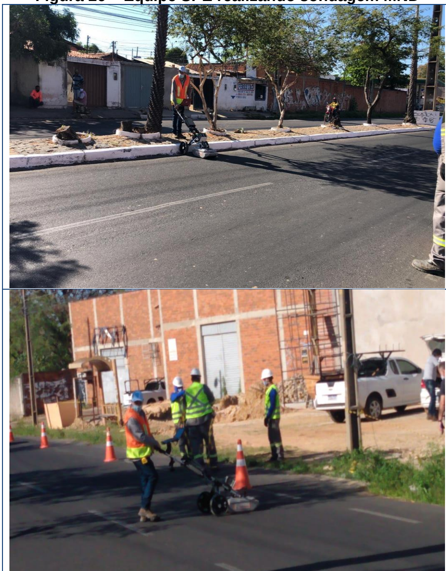
Figura 26 – Equipe SPE realizando sondagem MND
