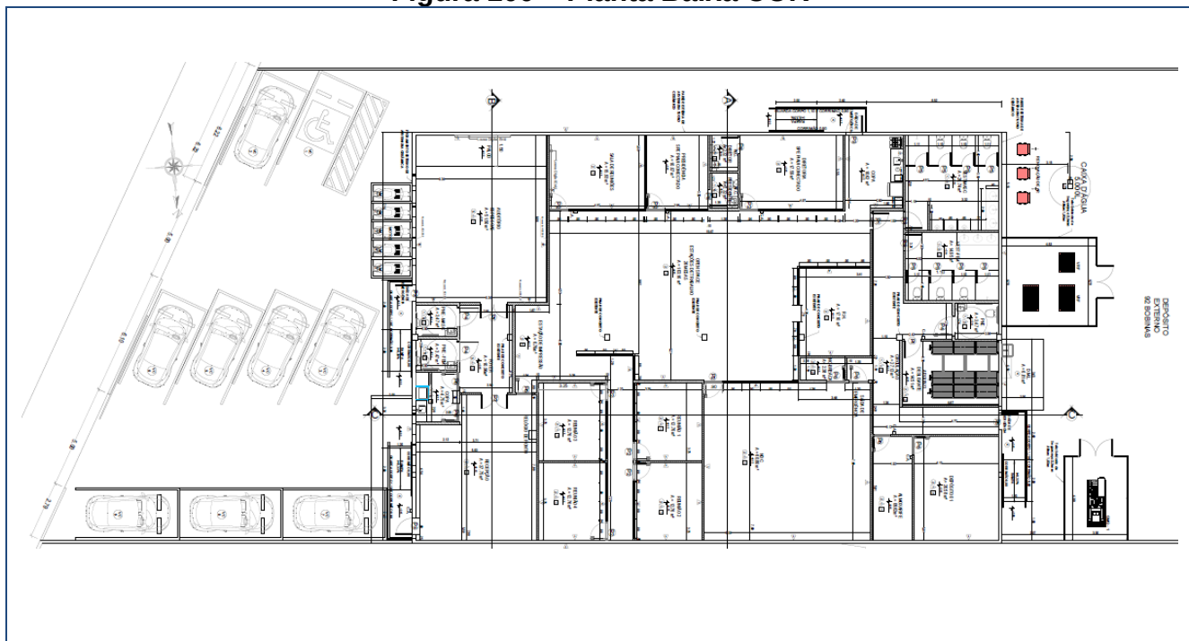
Figura 100 – Planta Baixa COR
