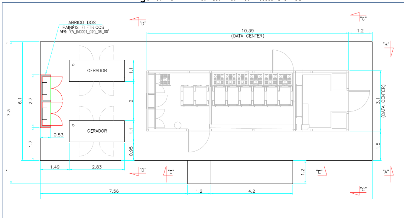
Figura 102 – Planta Baixa Data Center
