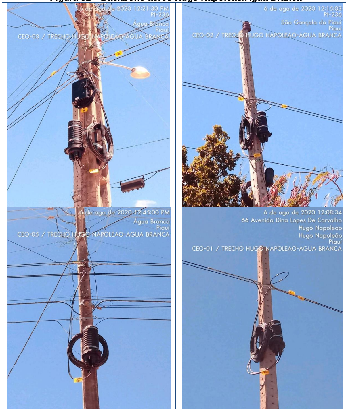
Figura 31 – Backbone aéreo Hugo Napoleão/Água Branca
