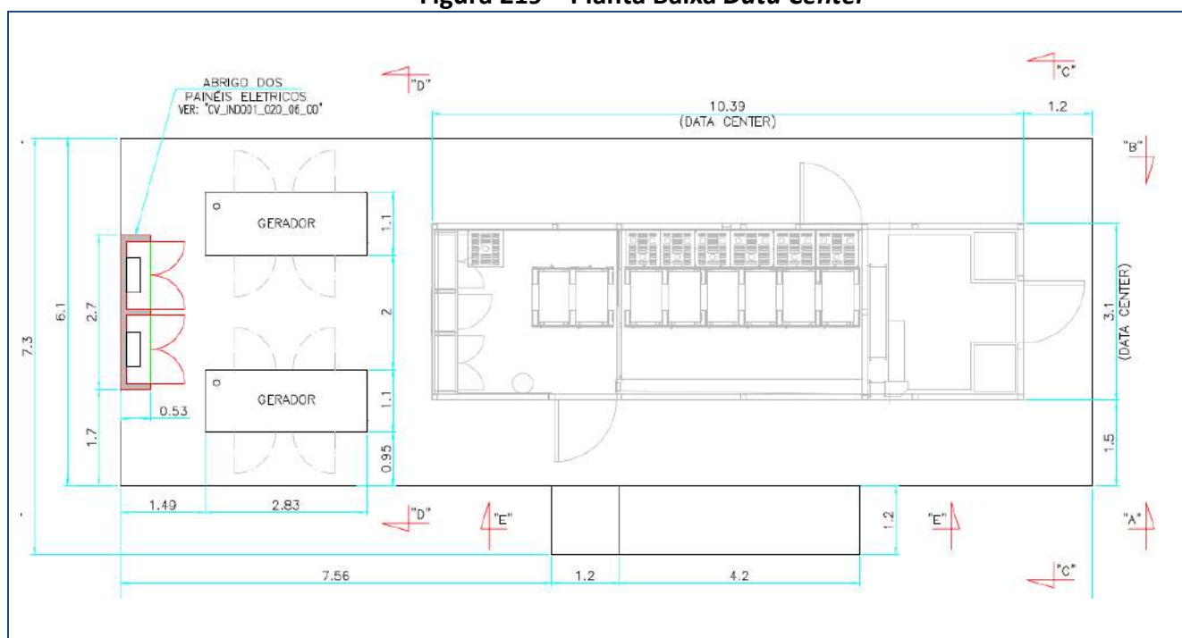
Figura 219 – Planta Baixa Data Center
