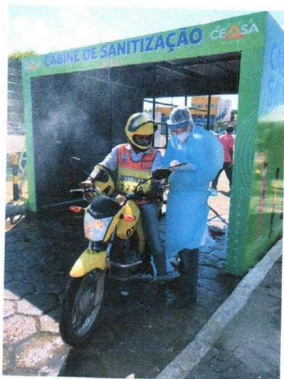
Fig. 11 – Instalação de Cabine Sanitária para motos e pedestres.
